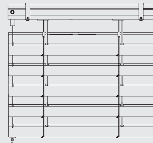
Obr. 2 - bočné vedenie v lanku
